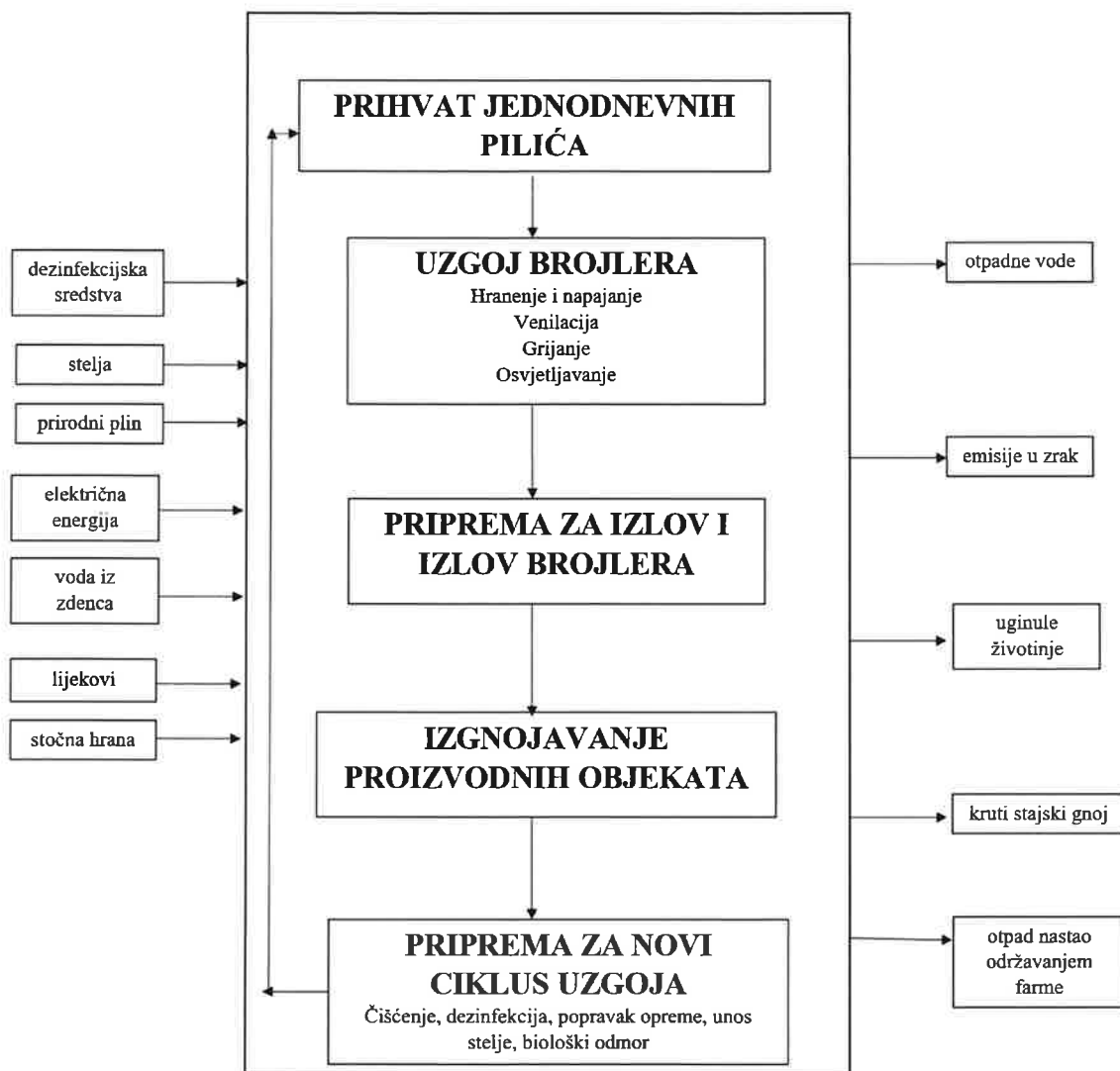
Prilog 2. Bok dijagram tehnološkog procesa na postojećem postrojenju za intenzivan uzgoj peradi Farma 9
